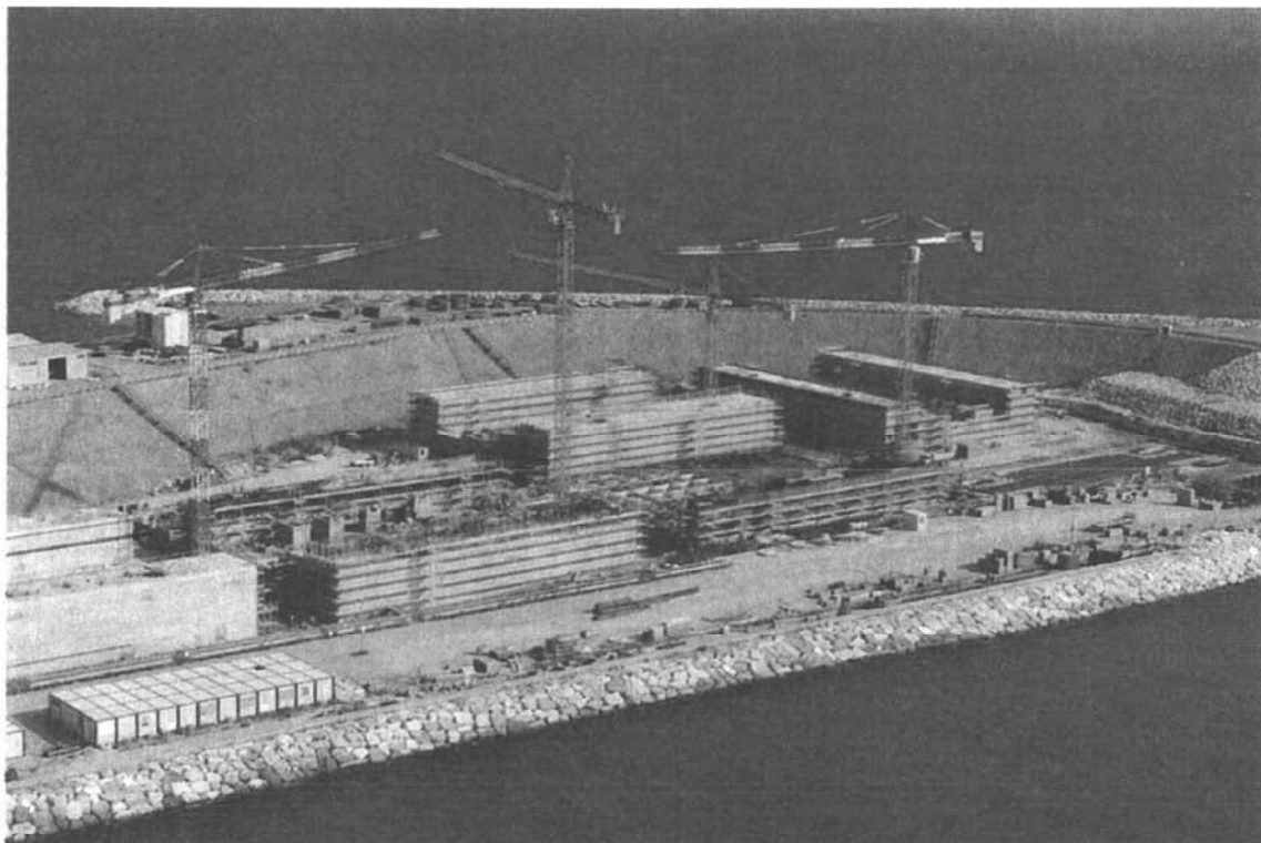
Bocca di Chioggia: il bacino del porto rifugio lato mare. Il bacino è stato messo all'asciutto e utilizzato come "tura" per la prefabbricazione dei cassoni di alloggiamento delle paratoie della barriera di Chioggia
